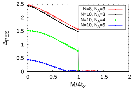
Entanglement gap
